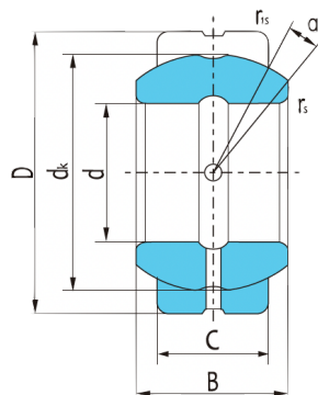
GEG...ES
