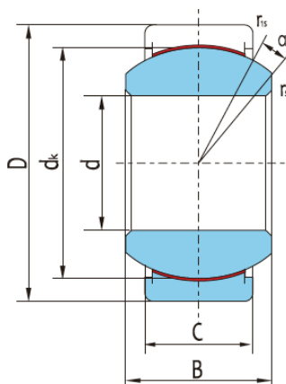
GEG...ET-2RS
