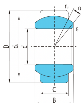
GEG...E
