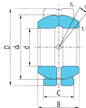
GEG...ES-2RS
